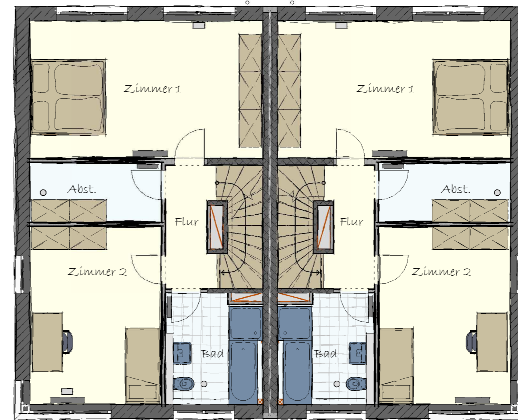
Obergeschoss Haus 206
