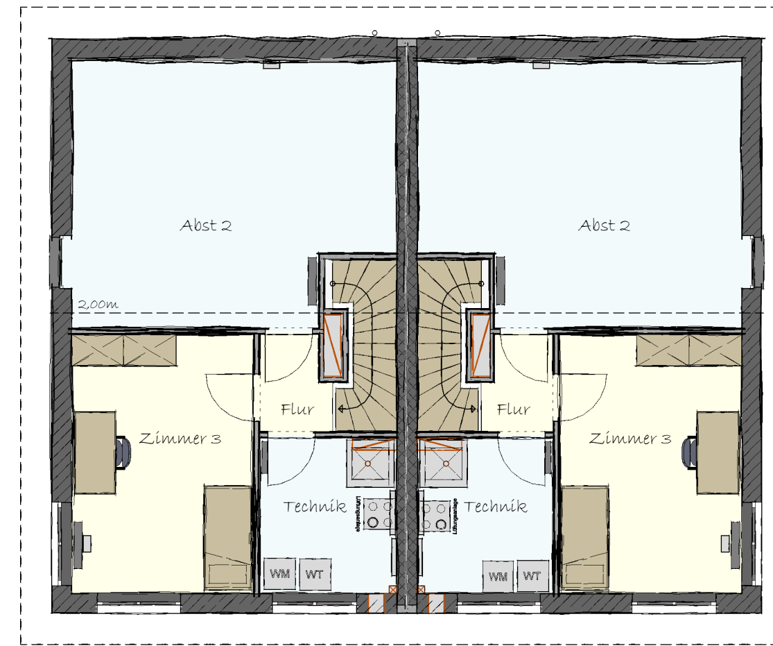
Dachgeschoss Haus 206
