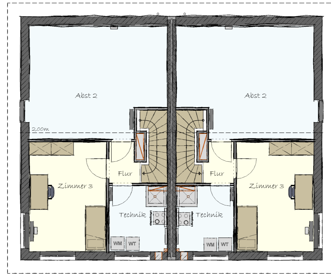
Dachgeschoss Haus 206
