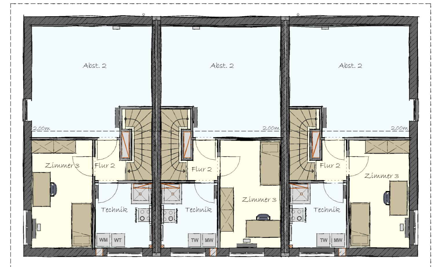
Dachgeschoss Haus 201
