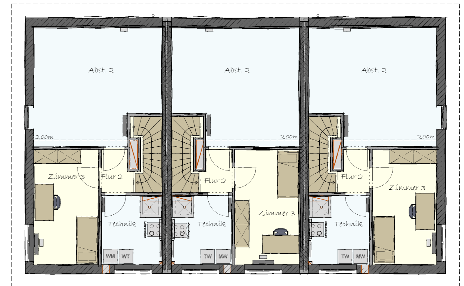
Dachgeschoss Haus 201
