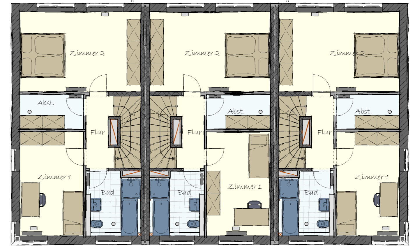
Obergeschoss Haus 201
